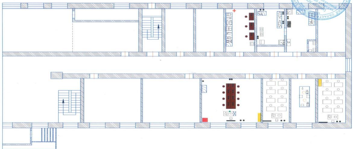
План застройки мастерской по компетенции "Стоматология ортопедическая", находящейся в г. Кемерово по ул. Николая Стровского, 10 этаж 1, площадь 131,1 м 2
