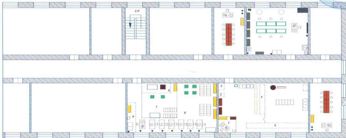
План застройки мастерской по компетенции "Фармацевтика", находящейся в г. Кемерово по ул. Николая Островского, 10 этаж 3, площадь 172,7 м 2
